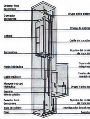
Ascensor hidráulico
