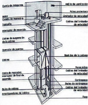
Ascensor eléctrico
